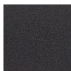
Nébuluse du graphite
